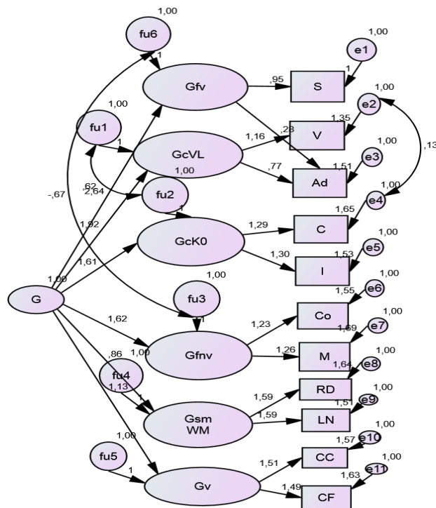
Figura 3. Estructura factorial de la adaptación argentina de WISC-IV según el modelo CHC.
